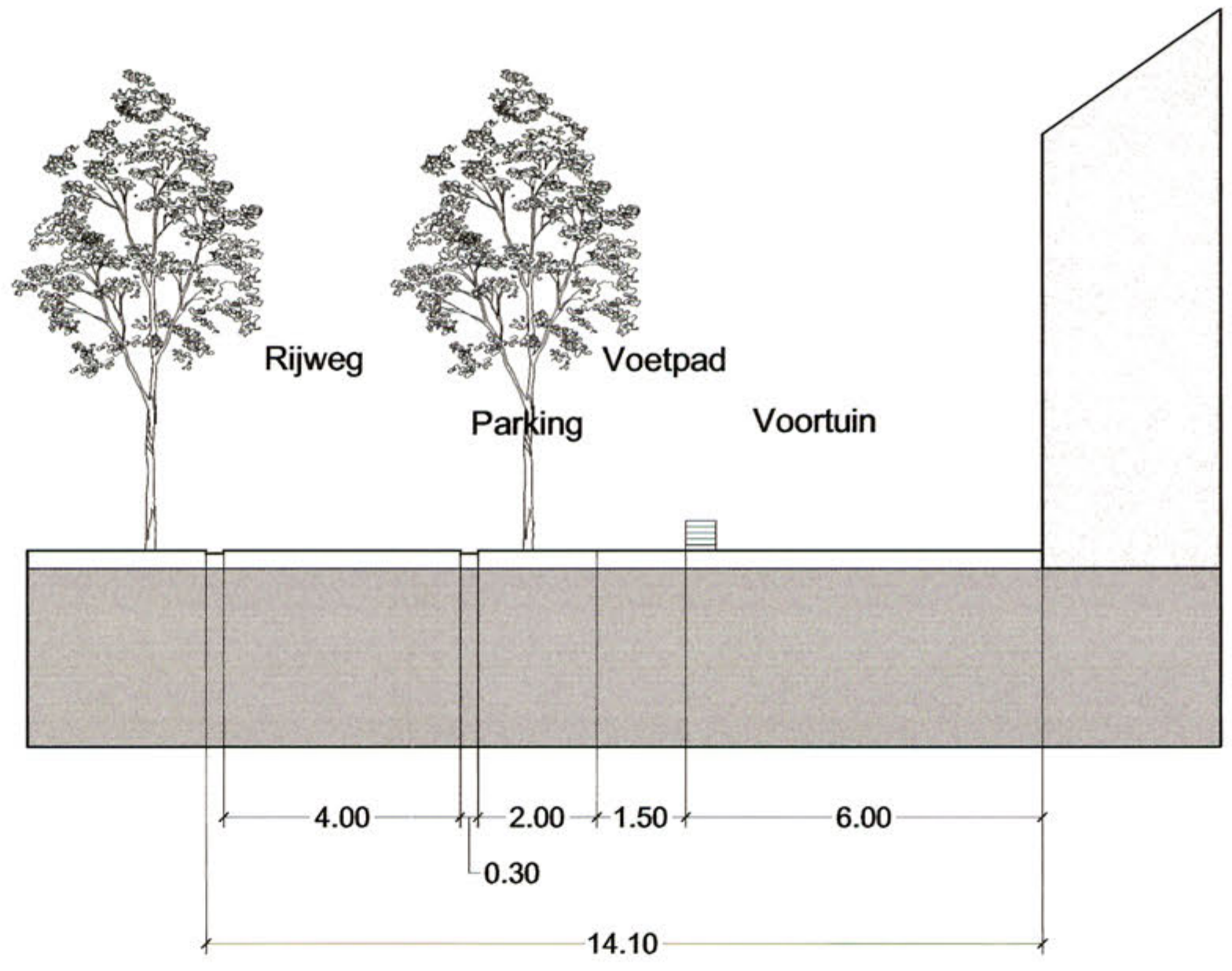
Snede AA', hoofdlaan, schaal 1/100
